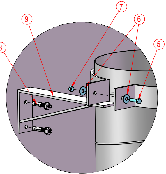
DETTAGLIO B
